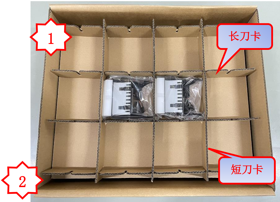
图二，将 PA4447 按照每层 12PCS，每箱 3 层的方式进行包装，同时在底层和每层的顶部放一块隔板，共 4 块隔板。
